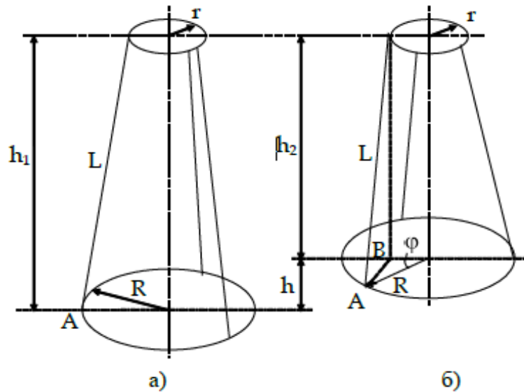
Рис. 3. Трифилярный подвес
